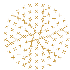
Gráfico 5 - Parte interna da orelha
