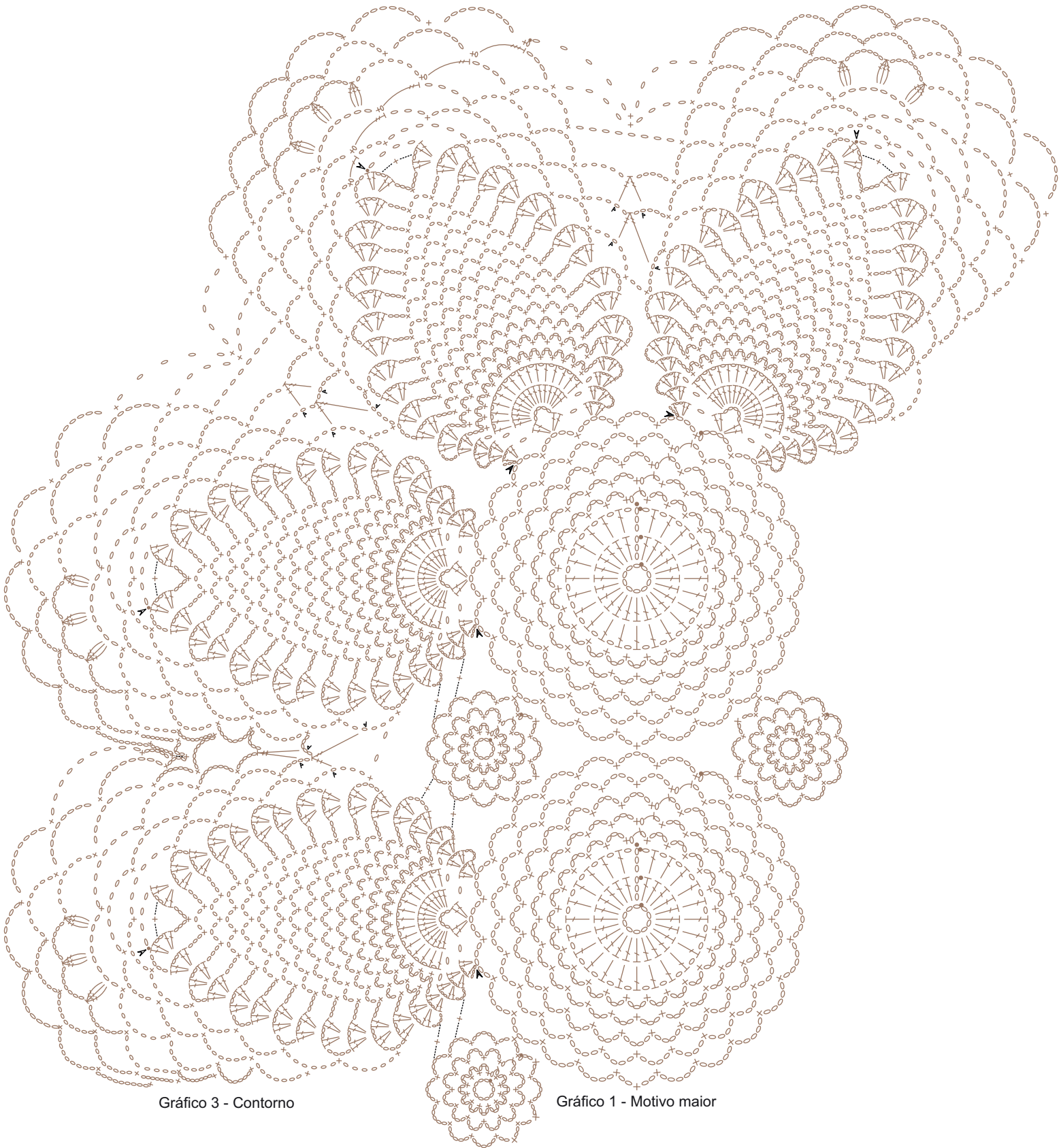
Gráfico 2 - Motivo menor
