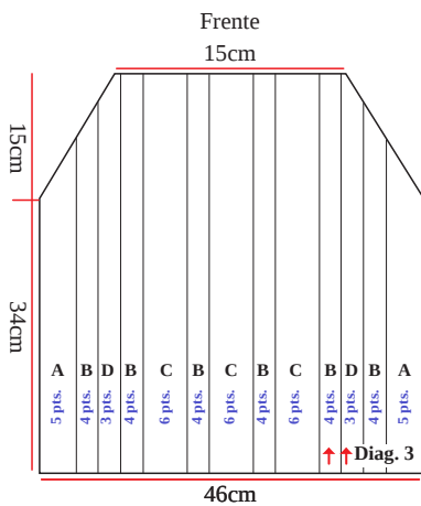
Esquema de medidas
