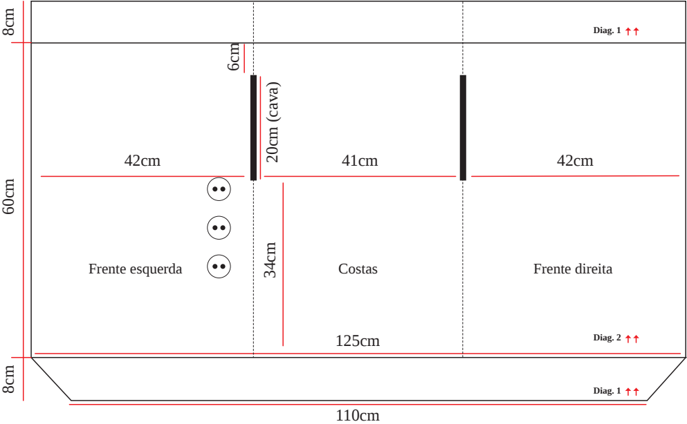
Esquema de medidas
