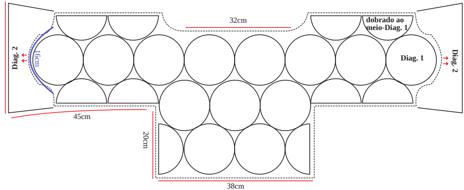
Esquema de medidas Costas = Frente
