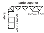
Gráfico 7 - Barrado das laterais e parte superior do pano
