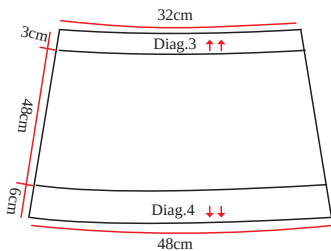
Esquema de medidas: Saia Parte da frente = parte atrás
