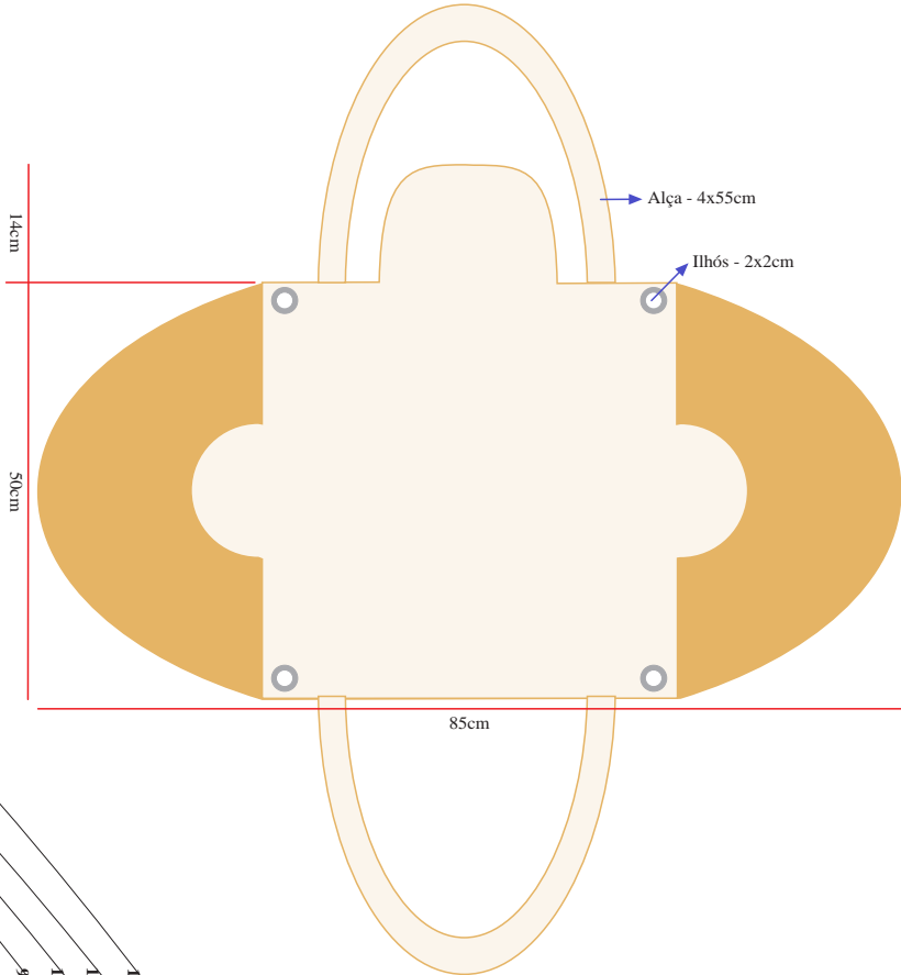
Esquema de medidas: Avesso da base da bolsa
