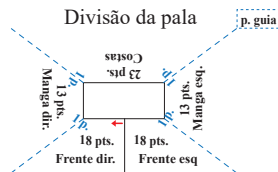
Esquema de medidas
