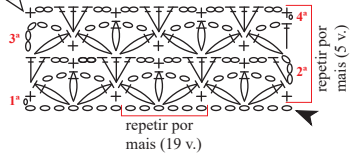
Diagrama 1 - Ponto fantasia (A)
