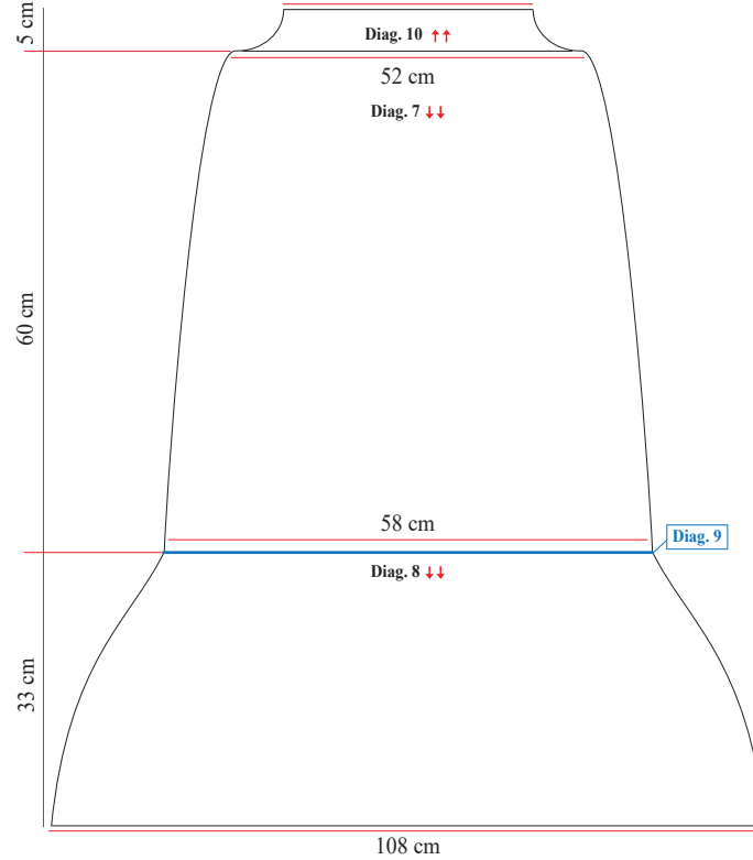
Saia Parte da frente = parte detrás 30 cm
