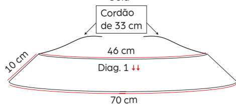
Esquema de medidas Gola
