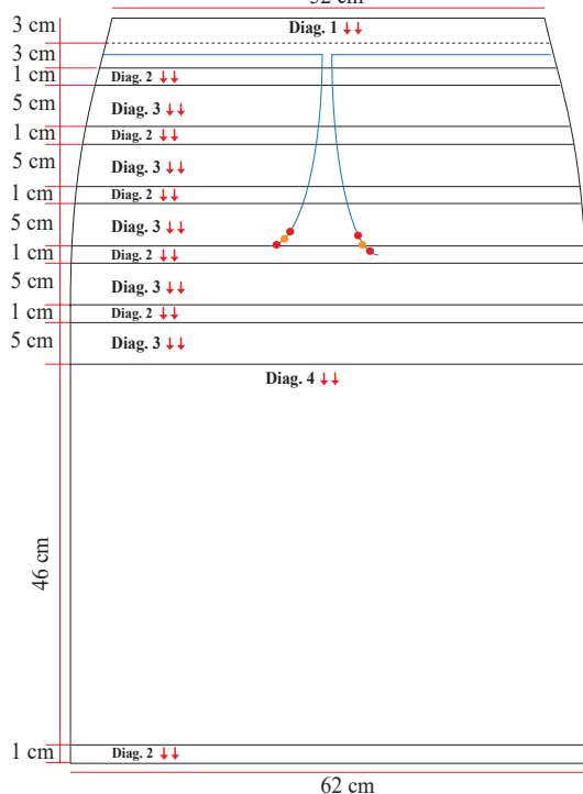
Esquema de medidas Parte detrás = parte da frente 52 cm
