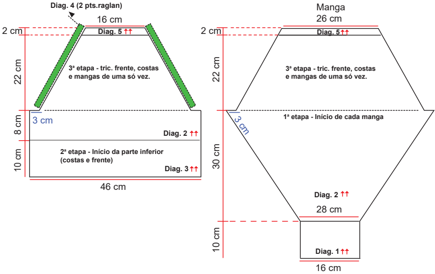
Esquema de medidas Costas=Frente
