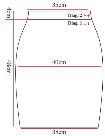
Esquema de medidas Parte da frente igual a parte atrás
